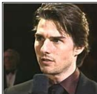
CNN
