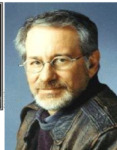
CNN
